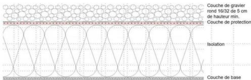
Image 1: Structure typique d'un toit en gravier
