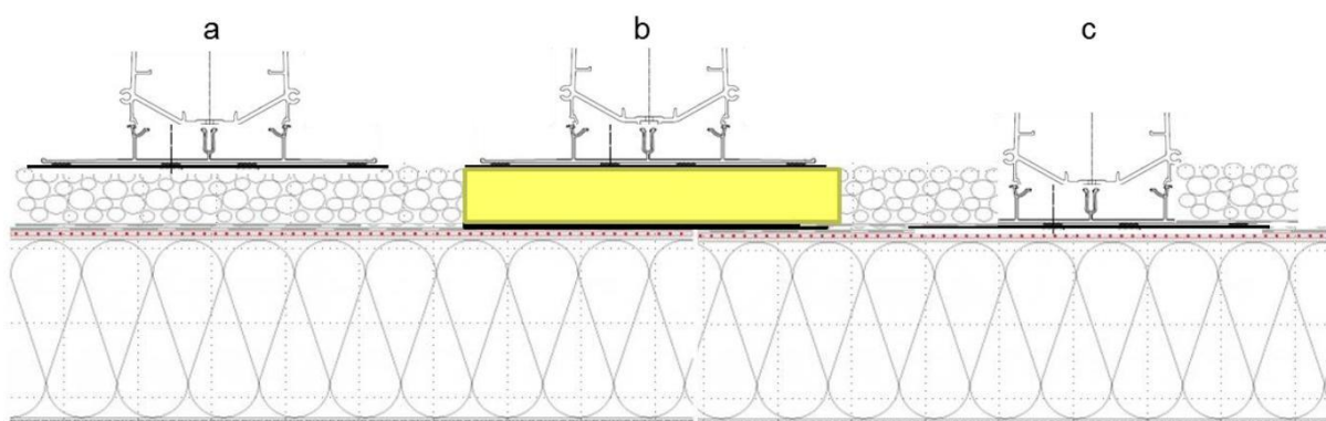
Image 2: Options MSP-FR sur toit en gravier
