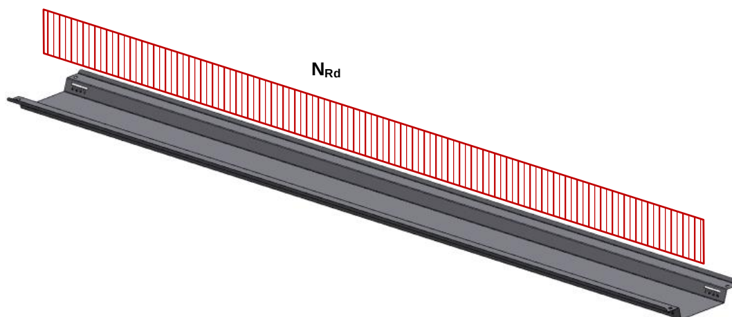
Abb. 5: MSP-FR-S-WD Darstellung der Lasteinwirkung
