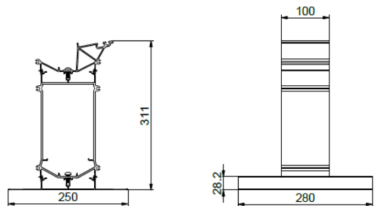
Abb. 13:Gründachstütze niedrig
