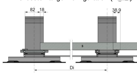
Grösste Längenkonfiguration (D i_max )
