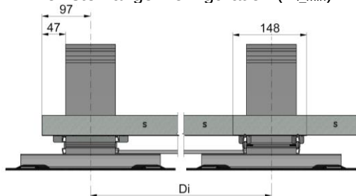
Kleinste Längenkonfiguration (D i_min )
