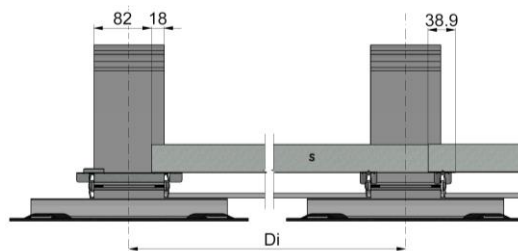
Configuration de la plus grande longueur (D i_max )
