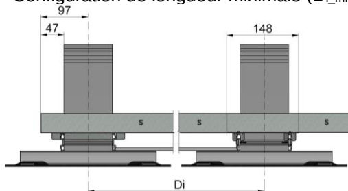
Configuration de longueur minimale (D i_min )
