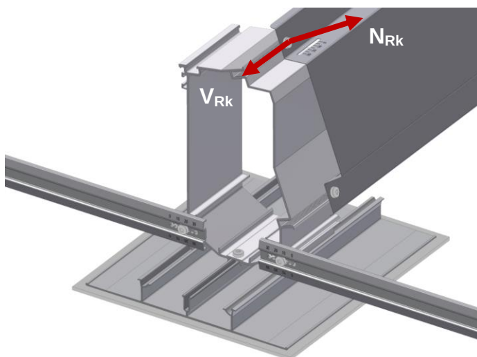
Illustration 5: vecteurs des résistances calculées pour la fixation du déflecteur de vent MSP-FR-S-WD
