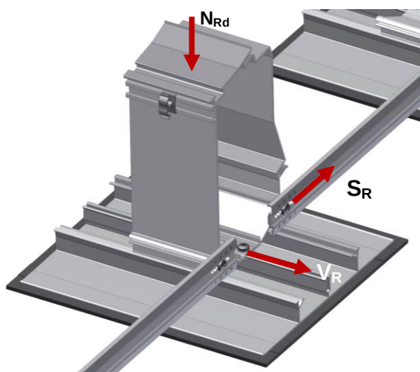
Illustration 2: vecteurs des résistances du support haut MSP-FR-S-SH
