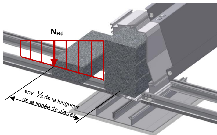
Illustration 3: vecteurs des résistances calculées de MSP-FR-EW-C
