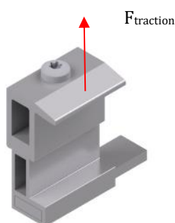
Illustration 10: vecteurs de résistance de la pince complémentaire haute MSP-FR-HC/B
