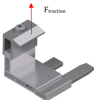
Illustration 9: vecteurs de résistance de la pince supplémentaire basse MSP-FR-LC/B
