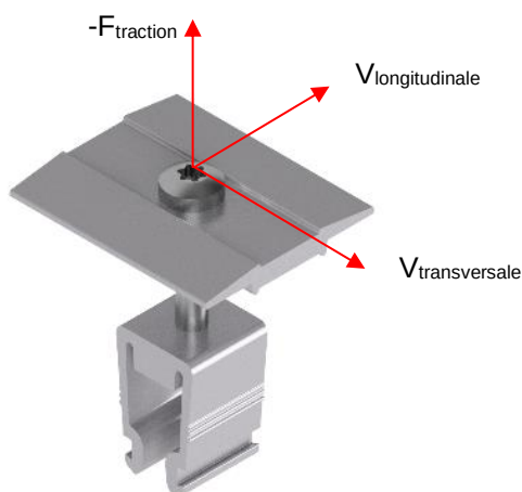
Illustration 7: vecteurs de résistance de la pince centrale MSP-PR-MC/G & MSP-PR-MCB/G
