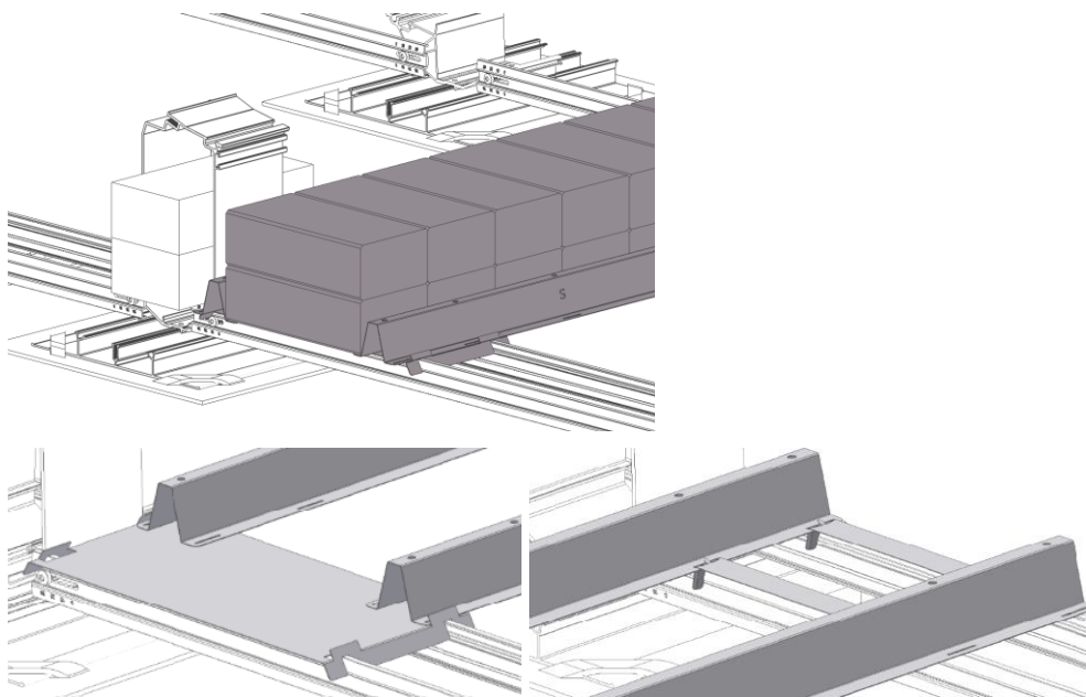
Illustration 4: Renforcement des barres de connexion
