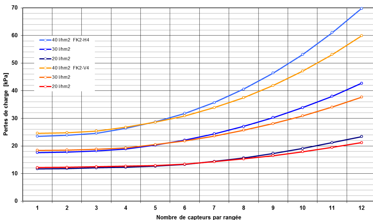
Pertes de charge des capteurs solaires FK2-H4 und FK2-V4 (rangée avec raccordement d'un côté et 2x30 cm de tuyau flexible DN16)
