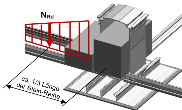
Abb. 3: Vektoren des Widerstands von MSP-FR-EW-C
