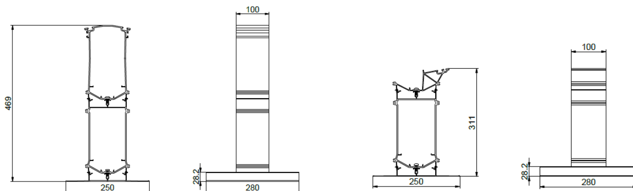
III. 12: Support pour toiture végétalisée haut
