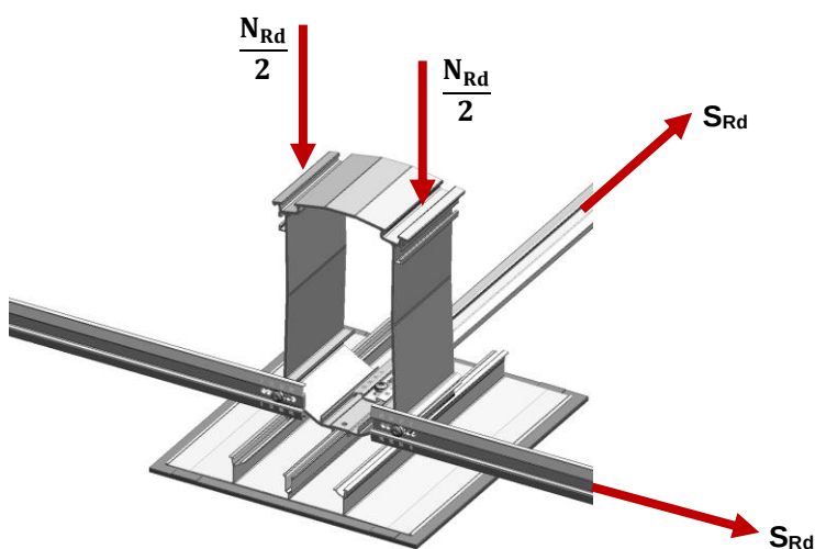
III. 2 : Vecteurs des résistances du support haut MSP-FR-EW-SH
