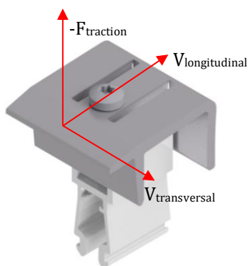
III. 7 : Vecteurs de résistance de la pince terminale
