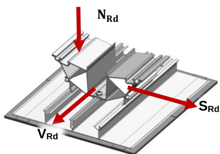
III. 1 : Vecteurs des résistances du MSP-FR-EW-SL8/SL10
