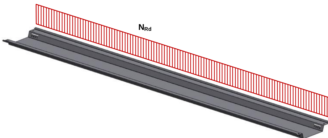
Fig. 5: Visualización MSP-FR-S-WD del efecto de la carga
