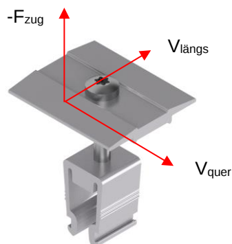
Fig. 6: Vectores de la resistencia de la abrazadera central
