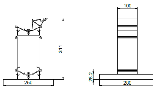
Fig. 13: Soporte de cubierta verde bajo
