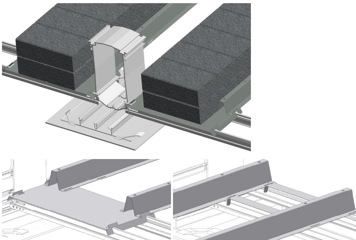
Fig. 4: Refuerzo de los raíles de conexión
