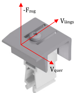
Fig. 7: Vectores de la resistencia de la abrazadera final
