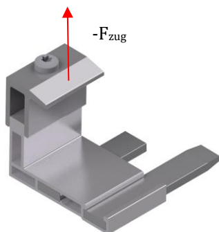
Fig. 8: Vectores de la resistencia de la abrazadera adicional baja
