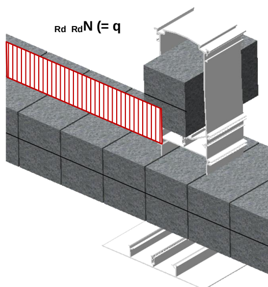
Fig. 11: Imagen del efecto de la carga sobre MSP-FR-EW-C
