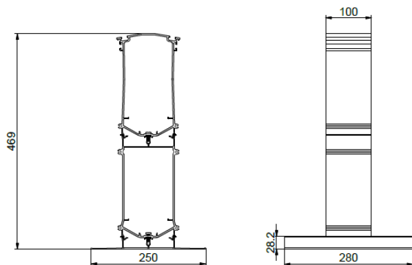
Fig. 12: Soporte de cubierta verde alto
