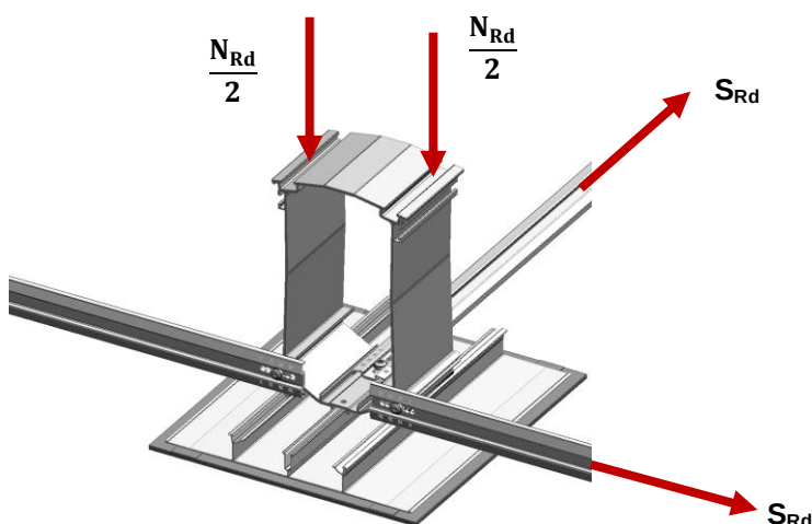
Fig. 2 Vectores de las resistencias del soporte alto MSP-FR-EW-SH
