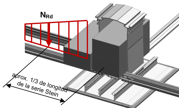
Fig. 3 Vectores de resistencia del carril de conexión MSP-FR-EW-C
