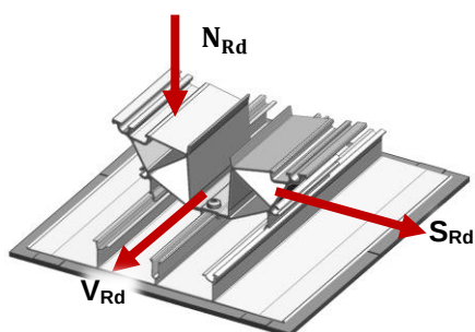
Fig. 1 Vectores de las resistencias del soporte bajo MSP-FR-EW-SL8/SL10
