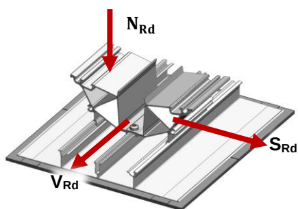
Fig.1 : Vectores de las resistencias del MSP-FR-EW-SL8/SL10
