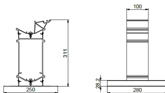
Fig. 13: Soporte de cubierta vegetal bajo
