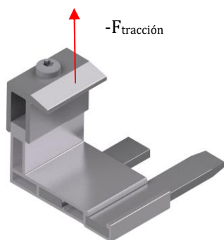
Fig. 8: Vectores de la resistencia del terminal adicional de la parte inferior
