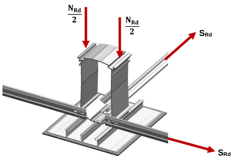
Fig.2 : Vectores de las resistencias del soporte alto MSP-FR-EW-SH
