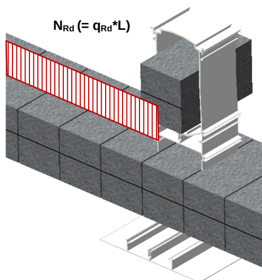
Fig. 11: Ilustración del efecto de la carga sobre MSP-FR-EW-C
