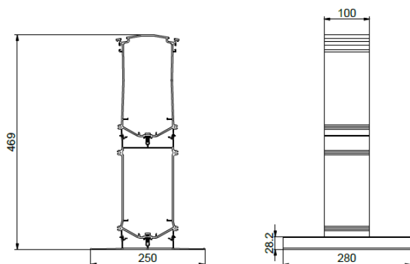
Fig. 12: Soporte de cubierta vegetal alto
