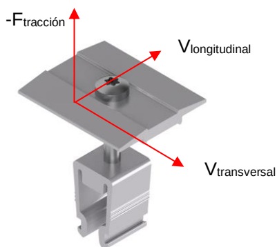
Fig. 6: Vectores de la resistencia del terminal central
