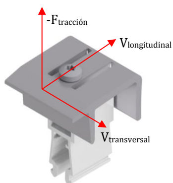
Fig. 7: Vectores de la resistencia del terminal final
