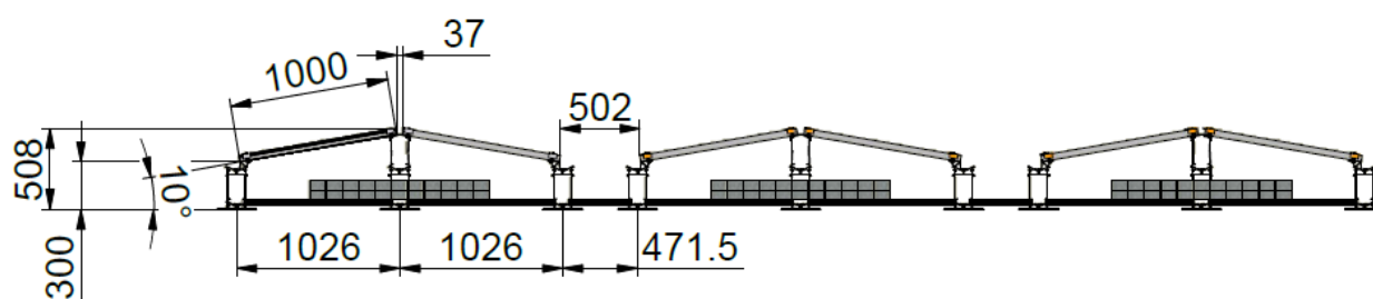
Fig. 14: Ejemplo - disposición en filas (sección) con módulos de 2000mm x 1000mm
