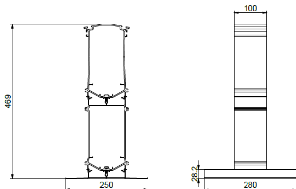
III. 12 : Support pour toiture végétalisée haut
