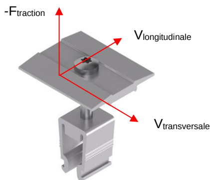
III. 6 : Vecteurs de la résistance de la borne centrale
