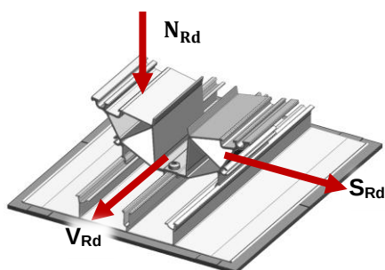
Rys.1 : Wektory rezystorów MSP-FR-EW-SL8/SL10
