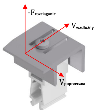
Rys. 7: Wektory rezystancji zacisku końcowego
