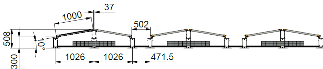
Rys. 14: Przykład - układ rzędów (sekcja) z modułami 2000 mm x 1000 mm
