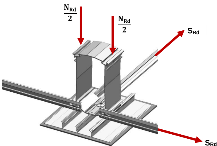
Rys.2 : Wektory rezystancji podpory wysokiej MSP-FR-EW-SH
