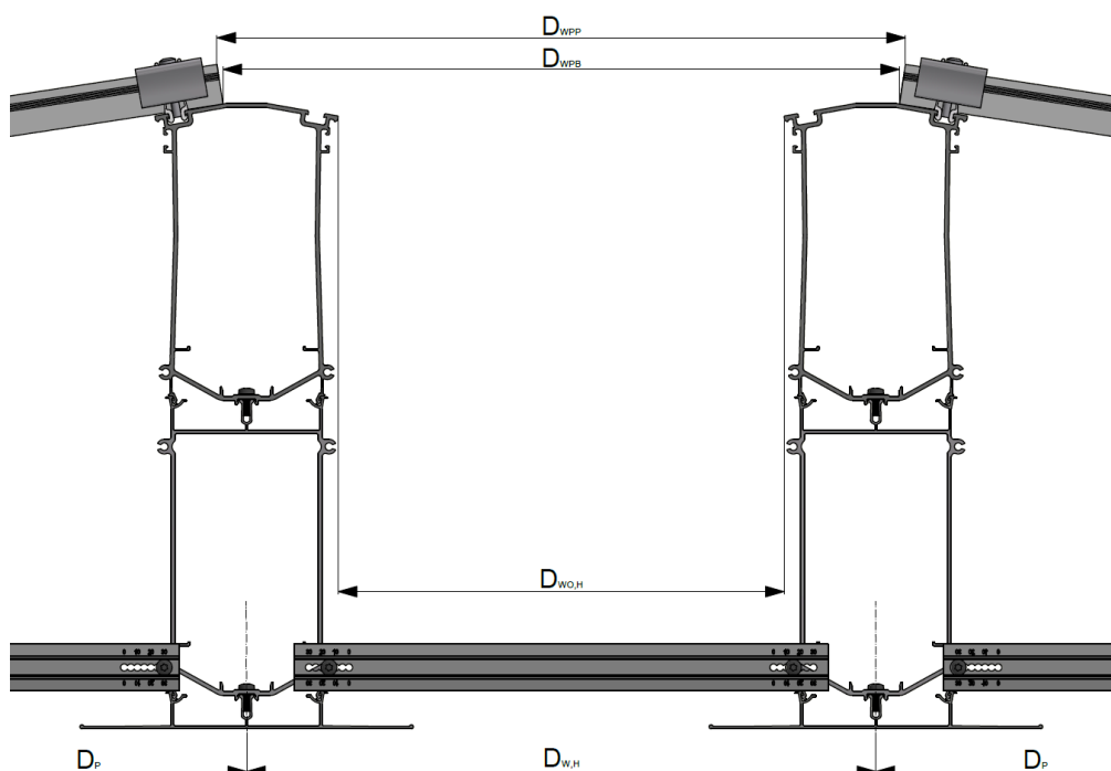
Rys. 16: Chodnik na grzbiecie
