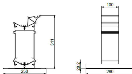
Rys. 13: Niski wspornik zielonego dachu
