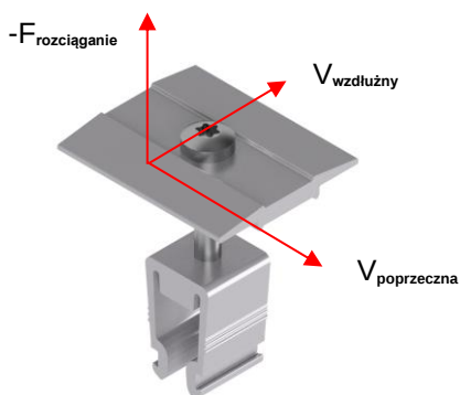
Rys. 6: Wektory rezystancji zacisku środkowego
