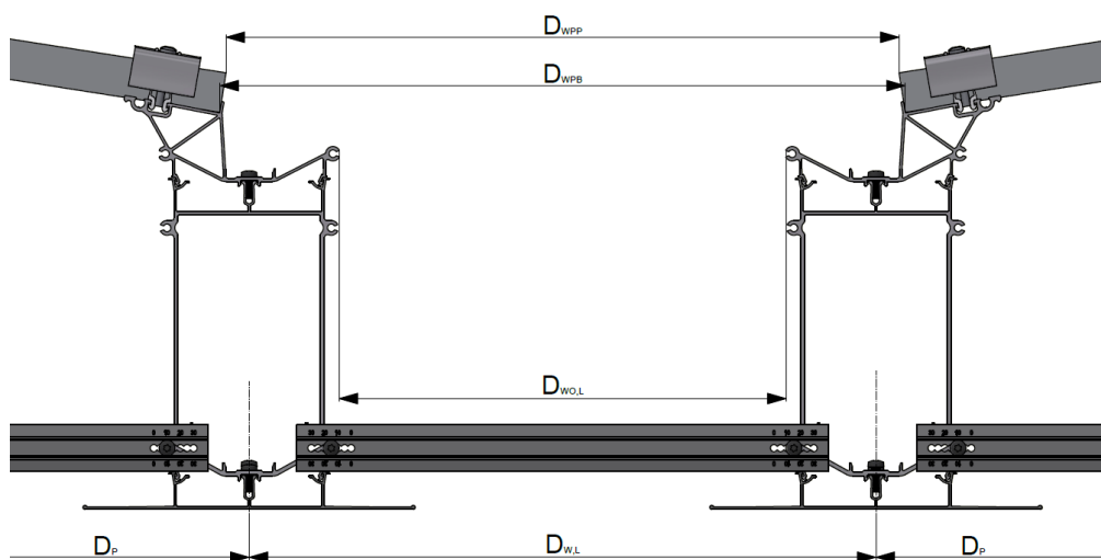
Rys. 16: Chodnik przy okapie
