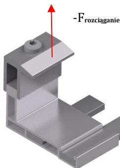
Rys. 8: Wektory rezystancji dodatkowego zacisku na dole
