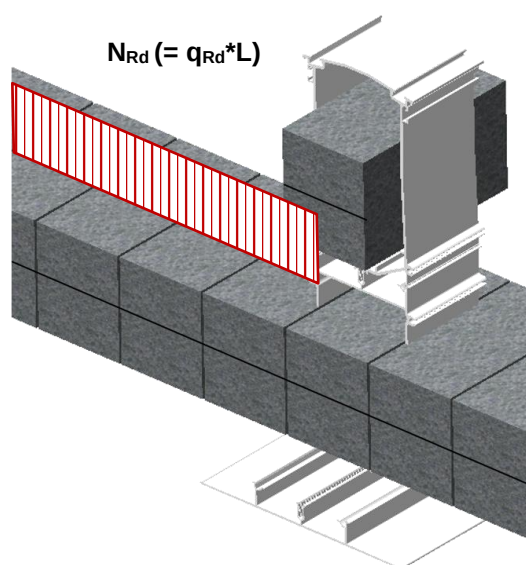
Rys. 11: Ilustracja wpływu obciążenia na MSP-FR-EW-C
