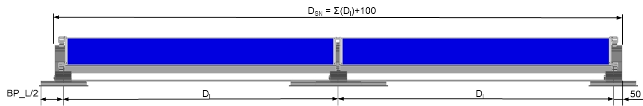
Dimensiones de los perfiles base
