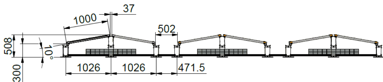
Fig. 14: Ejemplo - disposición en filas (sección) con módulos de 2000mm x 1000mm
