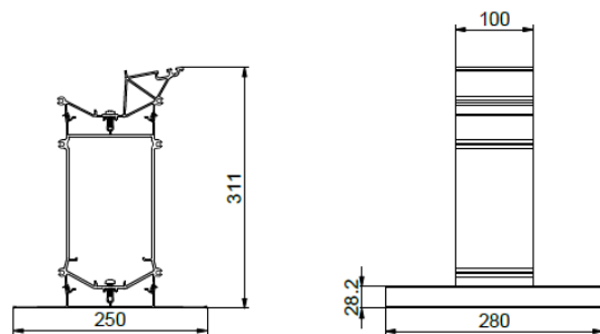
Fig. 13: Soporte de cubierta vegetal bajo
