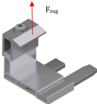
Abb. 8: Vektoren des Widerstands der Zusatzklemme tief
