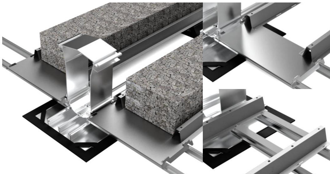
Abb. 5: Versteifung der Verbindungsschienen
