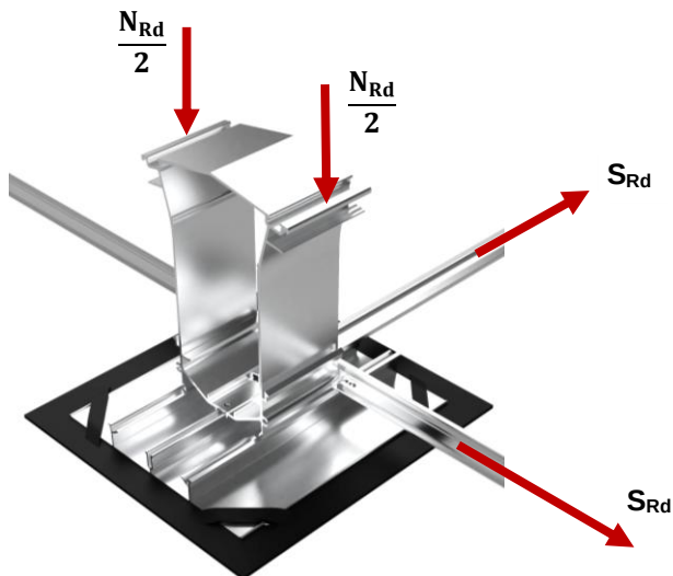
Abb. 2: Vektoren der Widerstände von MSP-FR-EW-SH90
