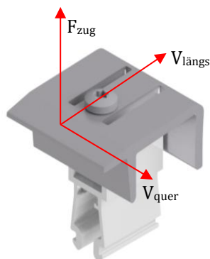
Abb. 7: Vektoren des Widerstands der Endklemme
