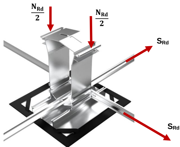
Abb. 3: Vektoren der Widerstände von MSP-FR-EW-SMH90
