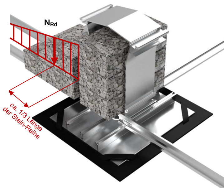
Abb. 4: Vektoren des Widerstands von MSP-FR-EW-C und MSP-FR-BF
