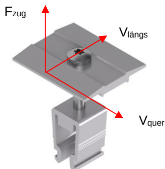
Abb. 6: Vektoren der Widerstände der Mittelklemme
