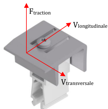
Fig.7 : Vecteurs de résistance de la pince terminale
