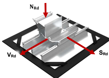
Abb. 2: Vektoren der Widerstände von MSP-FR-S-SL8/SL10
