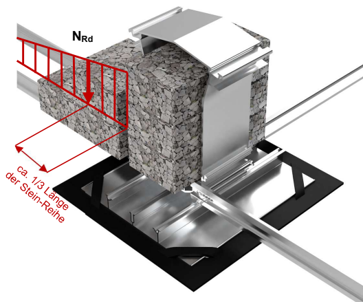
Abb. 5: Vektoren des Widerstands von MSP-FR-EW-C und MSP-FR-BF
