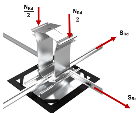
Abb. 4: Vektoren der Widerstände von MSP-FR-EW-SMH90
