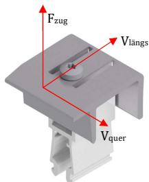
Abb. 8: Vektoren des Widerstands der Endklemme
