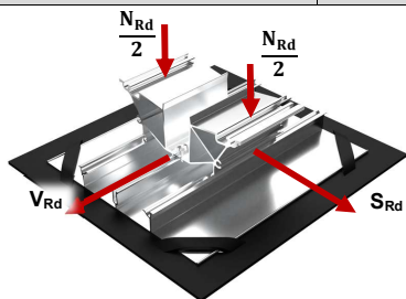
Abb. 1: Vektoren der Widerstände von MSP-FR-EW-SL8/SL10
