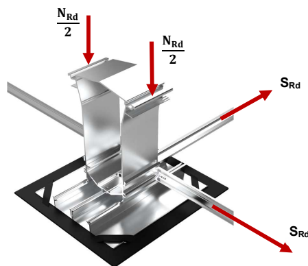
Abb. 3: Vektoren der Widerstände von MSP-FR-EW-SH90
