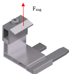
Abb. 9: Vektoren des Widerstands der Zusatzklemme tief
