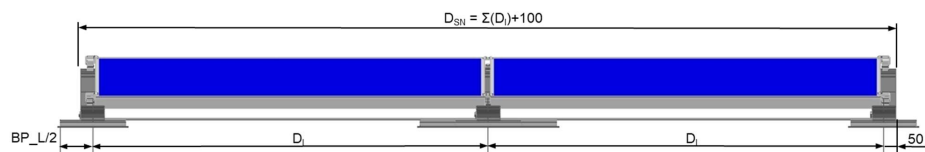
Abmessung Basisprofile
