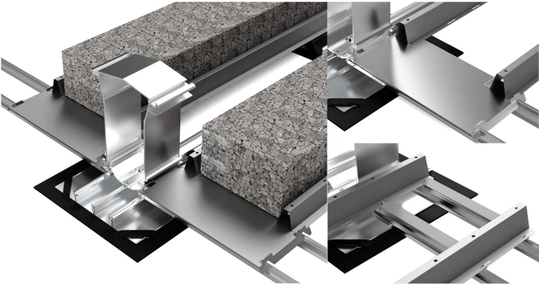
Abb. 6: Versteifung der Verbindungsschienen
