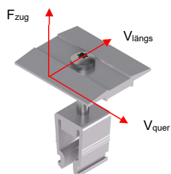
Abb. 7: Vektoren der Widerstände der Mittelklemme
