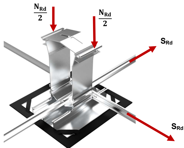
Fig.3 : Vecteurs des résistances du MSP-FR-EW-SMH90
