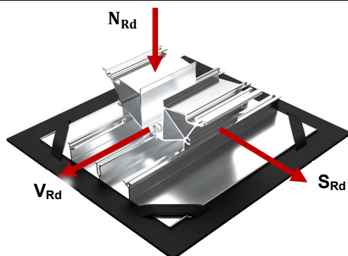
1 : Vecteurs des résistances des MSP-FR-EW-SL8/SL10
