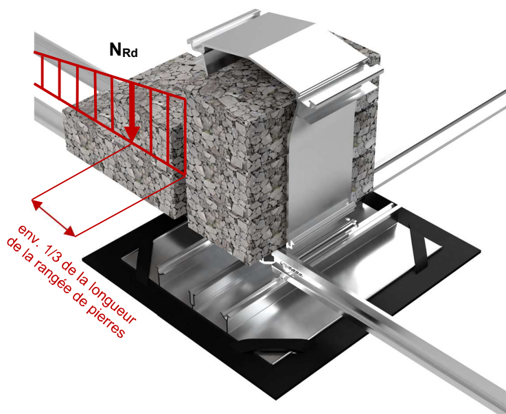
Fig.4 : vecteurs de résistance des MSP-FR-EW-C et MSP-FR-BF
