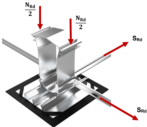
Fig.2 : Vecteurs des résistances du MSP-FR-EW-SH90
