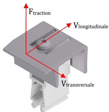
Fig.7 : Vecteurs de résistance de la pince terminale
