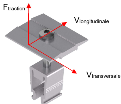
6 : Vecteurs des résistances de la pince centrale
